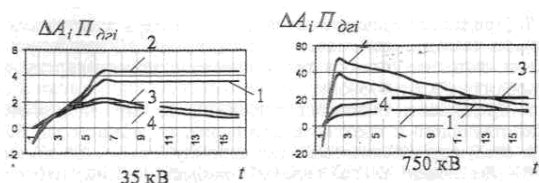
Рисунок 1 – Порівняння розвитку електричних мереж з використанням оптимального типоряду перерізів проводів: 1-втрати енергії в УПЛ; 2-втрати енергії в НПЛ; 3-дисконтований прибуток УПЛ; 4- дисконтований прибуток НПЛ
