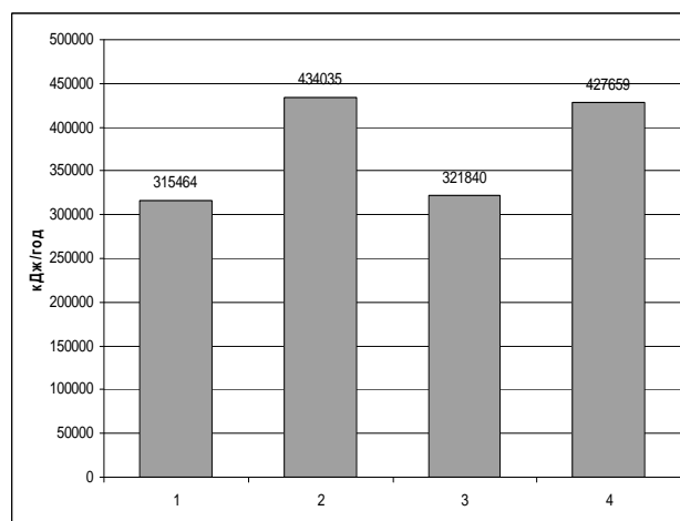
Рисунок 1 - Гістограма складових теплового балансу тваринницького приміщення: 1 - втрати тепла через огороження тваринницького приміщення; 2 - втрати тепла внаслідок вентиляції тваринницького приміщення; 3 - надходження тепла від тварин; 4 - надходження тепла від системи опалення
