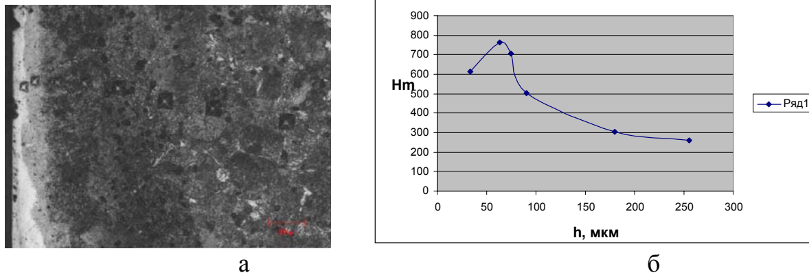
Рисунок 4 – Распределение микротвердости по глубине слоя при ЭЭЛ стали 40ХН2МЮА углеродом ( W_p = 0,9 Дж)
