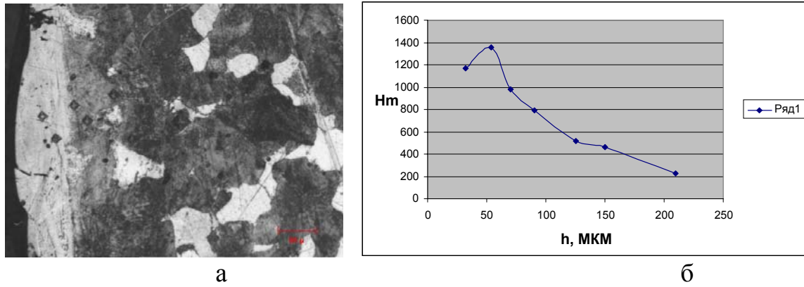
Рисунок 3 – Распределение микротвердости по глубине слоя при ЭЭЛ стали 38ХМЮА углеродом ( W_p = 0,9 Дж)
