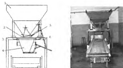
Рисунок 6 – Завантажувально-дозуючий пристрій: 1 - приймач насіння; 2 - заслінка; 3 - рама; 4 - дозуючий бункер; 5, 6 - механізми відкриття заслінок
