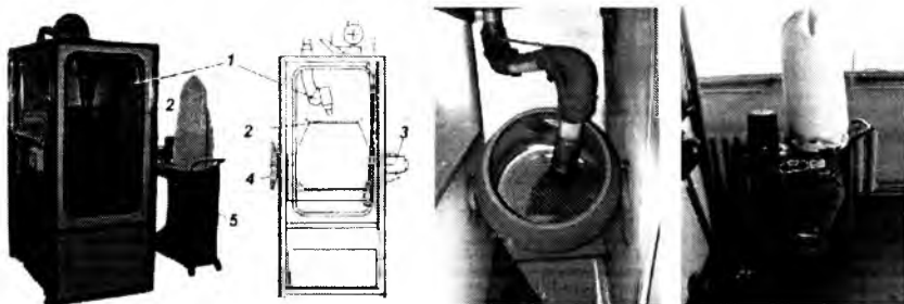
Рисунок. 1 – Установка вологого обезкрилення: 1 - кабінка з облаштуванням подання води і обдування повітрям; 2 - барабан-обезкрилювач; 3 - електродвигун; 4 - штурвал повороту барабана; 5 - фільтраційна установка
