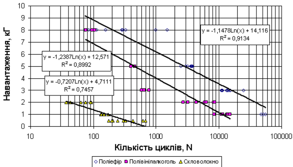
Рис. 6. Стійкість до дії багатocyклових навантажень 3-х типів ґраток
