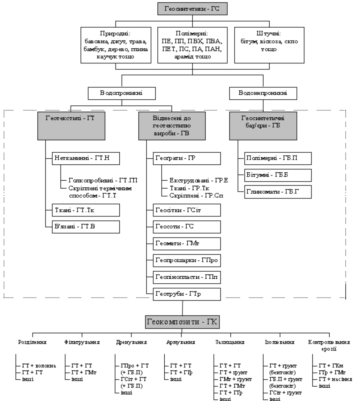
Рис. 1. Класифікація геосинтетиків за конструктивними параметрами
