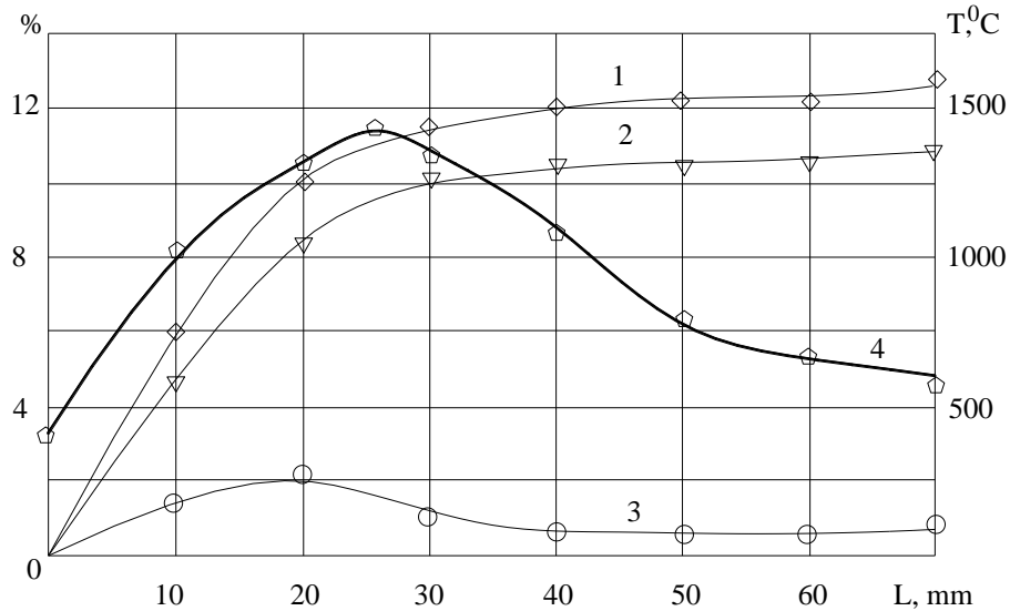
Рис. 1. Розподіл концентрацій та температур по довжині камери горіння: 1 – концентрація CO 2 при α = 1; 2 – CO 2 при α = 1,2; 3 – CO при α = 1,2; 4 – температура в топці
