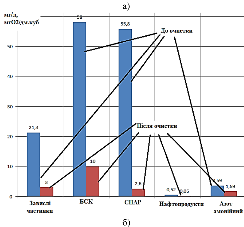
Рис. 6. Комбінована система електротехнологічної водоочистки (на прикладі підприємства малої металургії): А – зовнішній вигляд системи водоочистки, Б – ефективність функціонування комбінованої електротехнологічної очистки стічних вод
