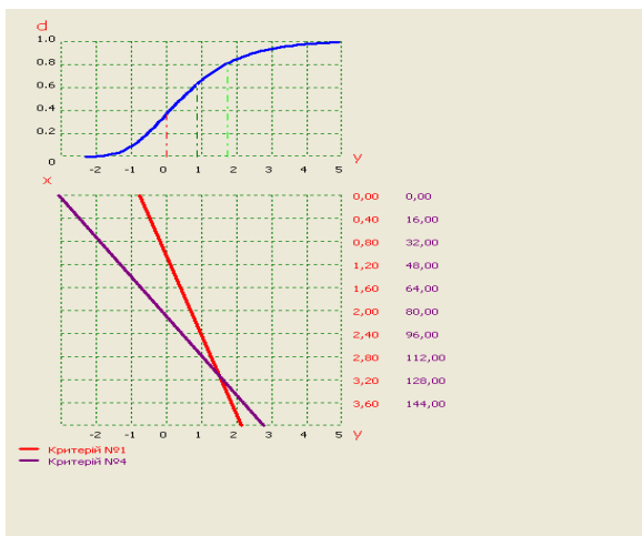
Рис. 1.а. Номограма худ для показників розрахункового розривального навантаження та ступеня білості
