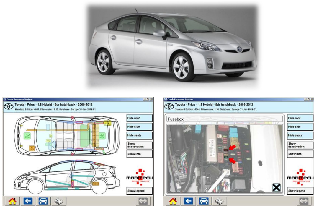
Рис. 6. Місце розташування АКБ в автомобілі Toyota Prius та порядок відключення системи
