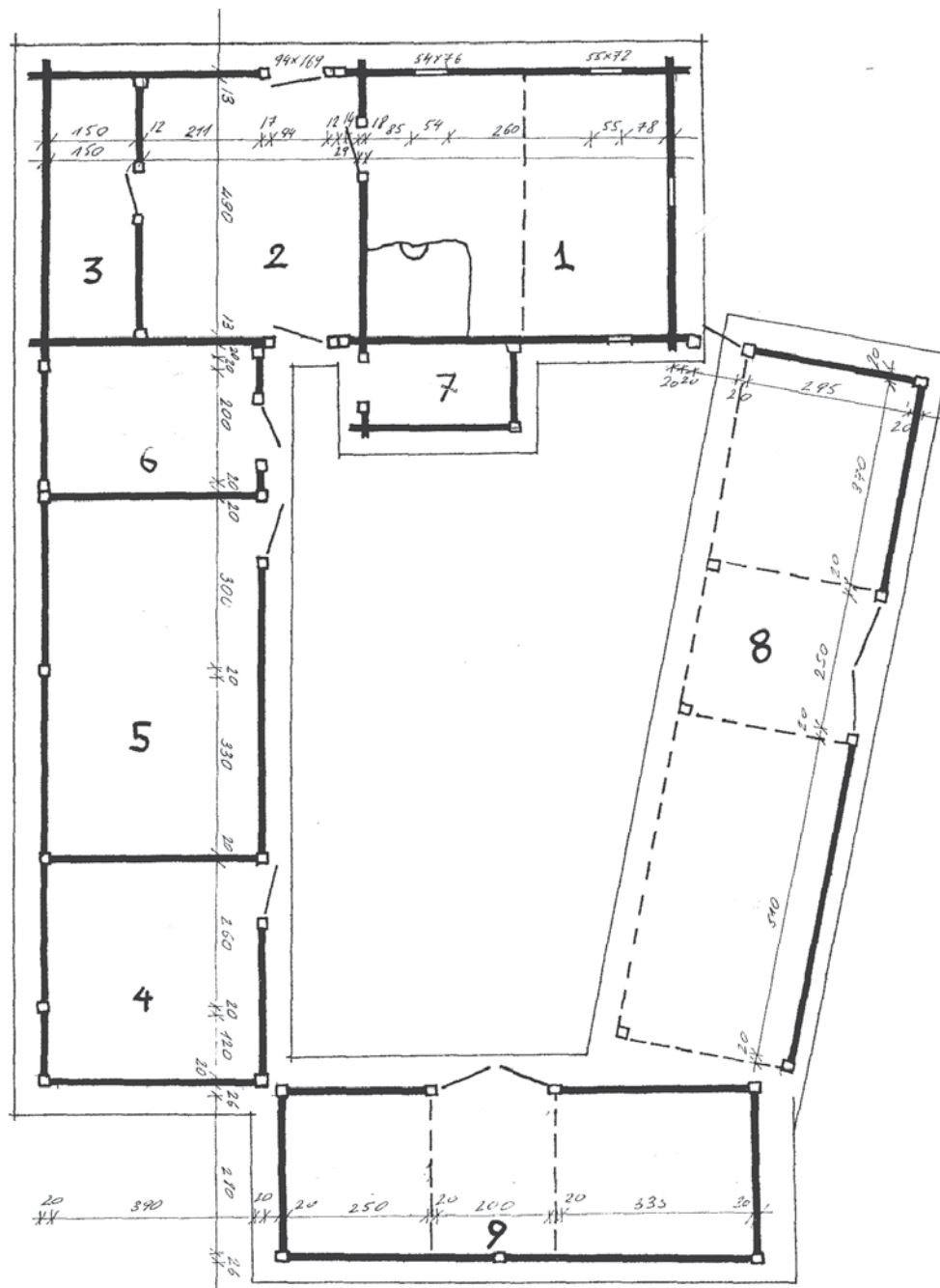
Рис. 9. "Підварок" кінця XIX ст. у с. Піщаному Камінь-Каширського р-ну Умовні позначки: 1 – хага; 2 – сіни; 3 – комора; 4 – хлів для корів; 5 – хлів для коней; 6 – хлівець для свиней; 7 – пукліт; 8 – шопя-навіс; 9 – клуня
