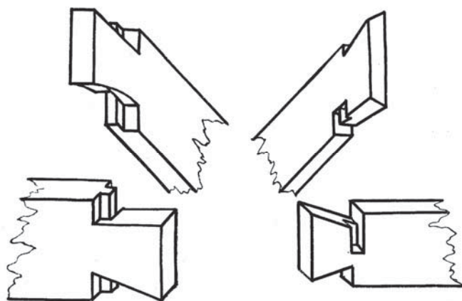
Рис. 7. Кутові врубки типу "риб'ячий хвіст" з прихованим зубом на Підляшші (за С. Стацак)
