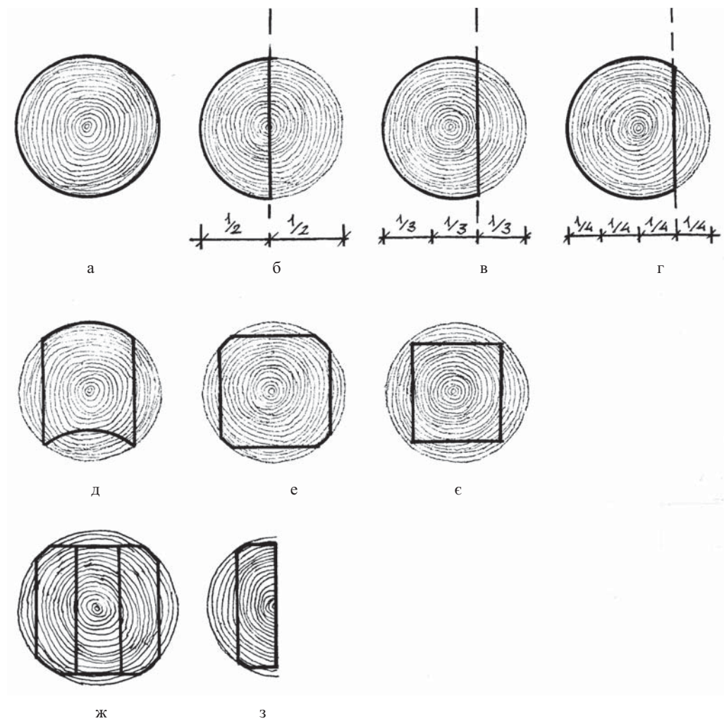
Рис. 1. Будівельна деревина
