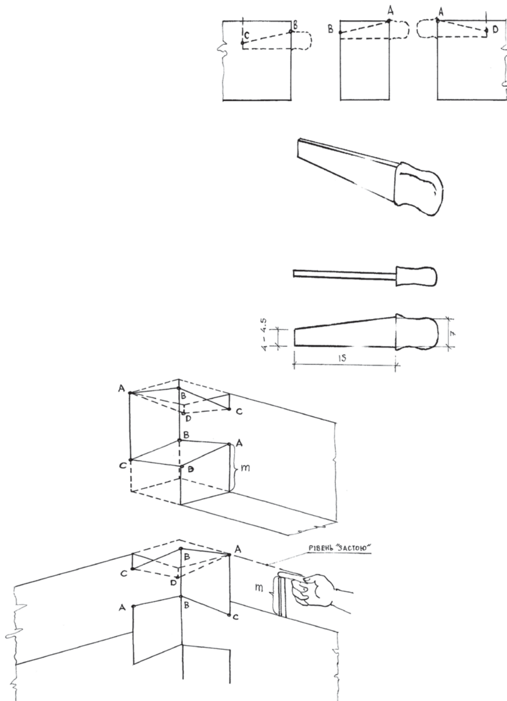
Рис. 3. Влаштування односторонньої врубки типу "риб'ячий хвіст"
