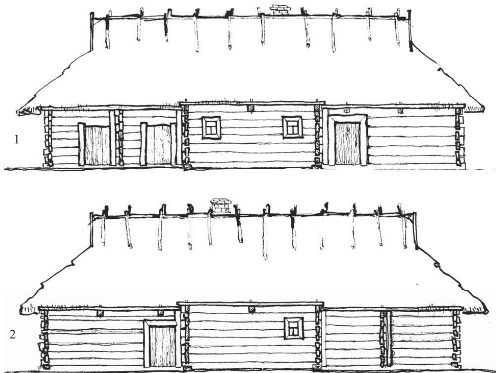
Рис. 11. Хага середини ХІХ ст. у с. Здомишлі Ратнівського р-ну 1 – головний фасад; 2 – тильний фасад
