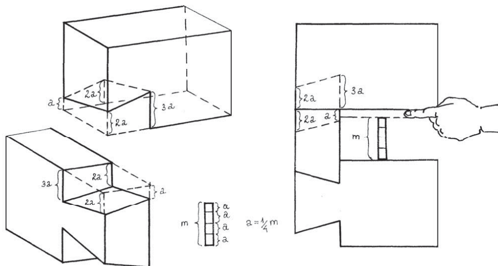
Рис. 2. Влаштування двосторонньої врубки типу “риб’ячий хвіст” без лишку
