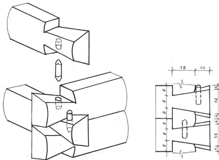
Рис. 8. Кутова врубка типу “риб’ячий хвіст” з випусками торців
