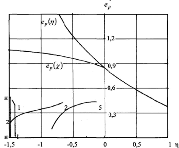
Рисунок 4. – Діаграма пластичності сталі 20Х і шляхи деформування небезпечних областей при вдавлюванні шліцьового штампа
