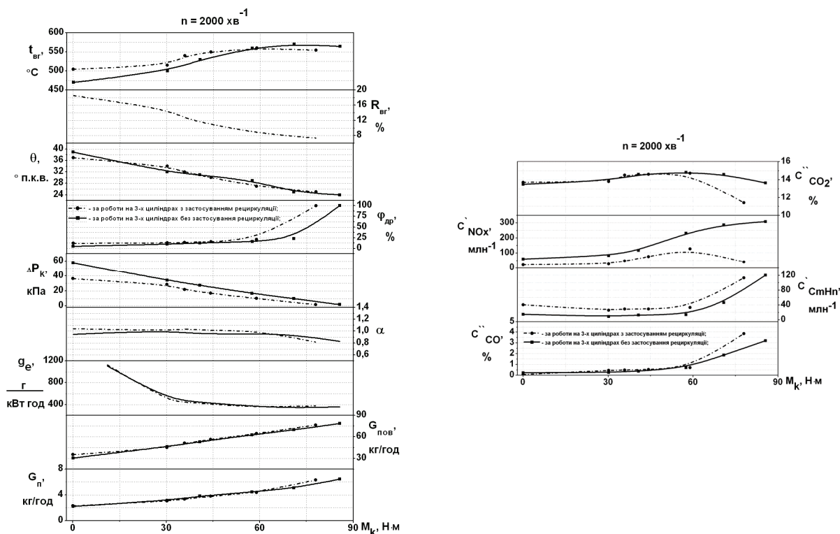
Рисунок 5 – Залежності показників двигуна 6C9,5/6,98 від навантаження
