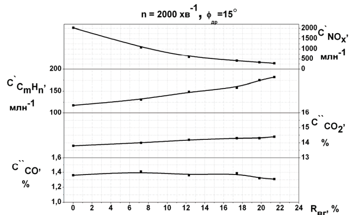
Рисунок 3 – Вплив коефіцієнта рециркуляції на концентрації шкідливих речовин з відпрацьованими газами двигуна 6C9,5/6,98
