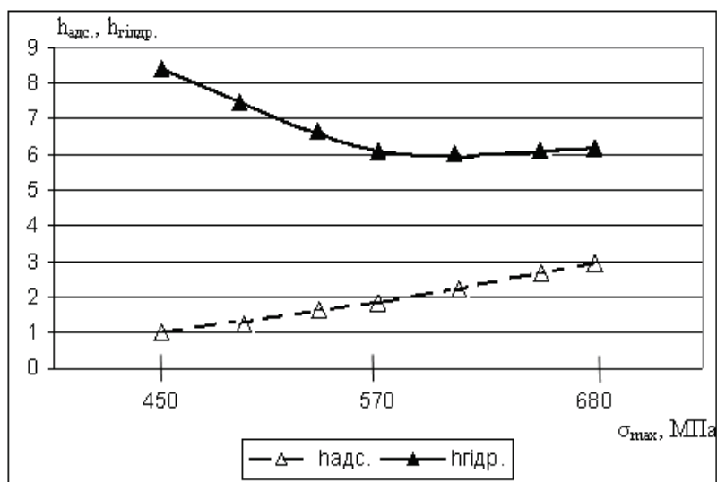
Рисунок 4. – Кінетика формування гідродинамічної ( h_{\text{гiдp.}} ) та негідродинамічної ( h_{\text{адс.}} ) складової товщини мастильного шару
