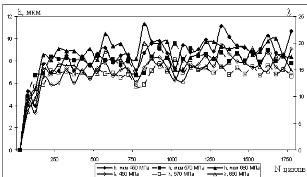
Рисунок 1. –Формування товщини мастильного шару (h) та режим мащення в контакті (λ) при напруженні
