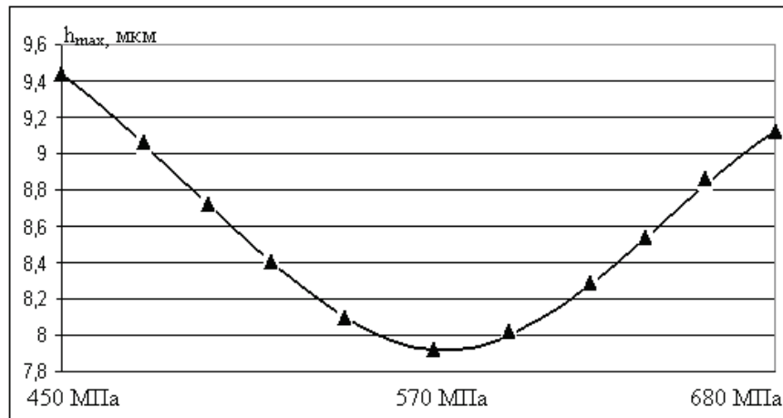
Рисунок 2. –Формування максимальної товщини мастильного шару ( h_{max} ) у залежності від навантаження ( \sigma_{max} )
