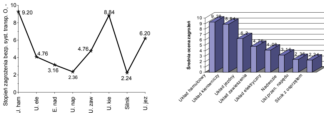
Rys. 3. Średnie wartości ocen zagrożenia bezpieczeństwa systemu transportowego, O , jakie stwarza uszkodzenie układów autobusów międzymiastowych i miejskich
