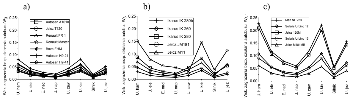
Rys. 5. Wartości wskaźnika W_3 oceny poziomu zagrożenia działania wynikające z uszkodzenia układu autobusów: a) międzymiastowych PKS Krosno, b) miejskich MZK Bydgoszcz, c) miejskich MPK Rzeszów
