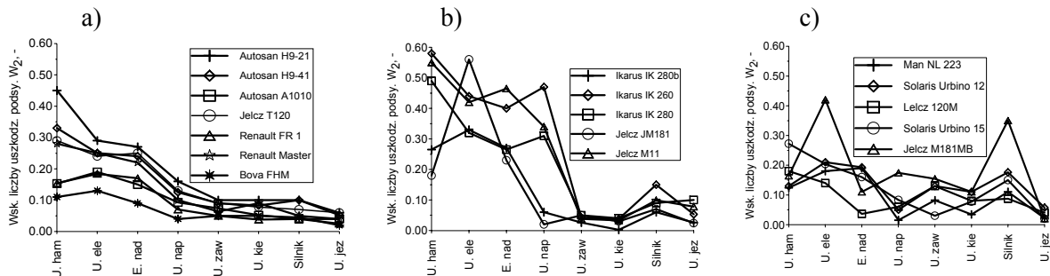
Rys. 2. Wartości wskaźnika W_2 liczby uszkodzonych układów autobusów: a) międzymiastowych PKS Krosno, b) miejskich MZK Bydgoszcz, c) miejskich MPK Rzeszów
