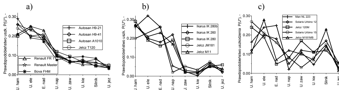
Rys. 4. Wartości prawdopodobieństwa wystąpienia uszkodzenia układów autobusów P(W^*) : a) międzymiastowych PKS Krosno, b) miejskich MZK Bydgoszcz, c) miejskich MPK Rzeszów
