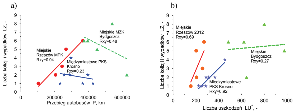
Rys. 7. Zależności liczby kolizji i wypadków autobusów międzymiastowych i miejskich od: a) przebiegu, b) liczby uszkodzeń.
