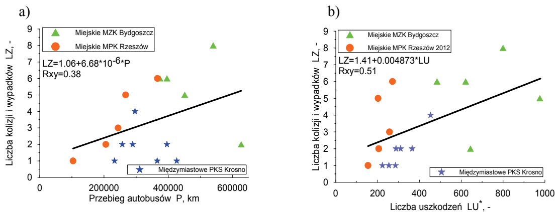
Rys. 8. Zależności liczby kolizji i wypadków autobusów międzymiastowych i miejskich od: a) przebiegu, b) liczby uszkodzeń.
