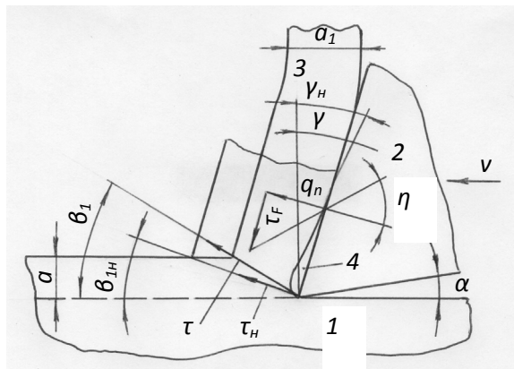
Рисунок 1 – Схема процесу низькошвидкісного вільного ортогонального різання
