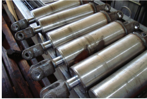
Рисунок 7 – Гідроциліндри Ц-100, виготовлені з використанням деформуюче-різального протягування
