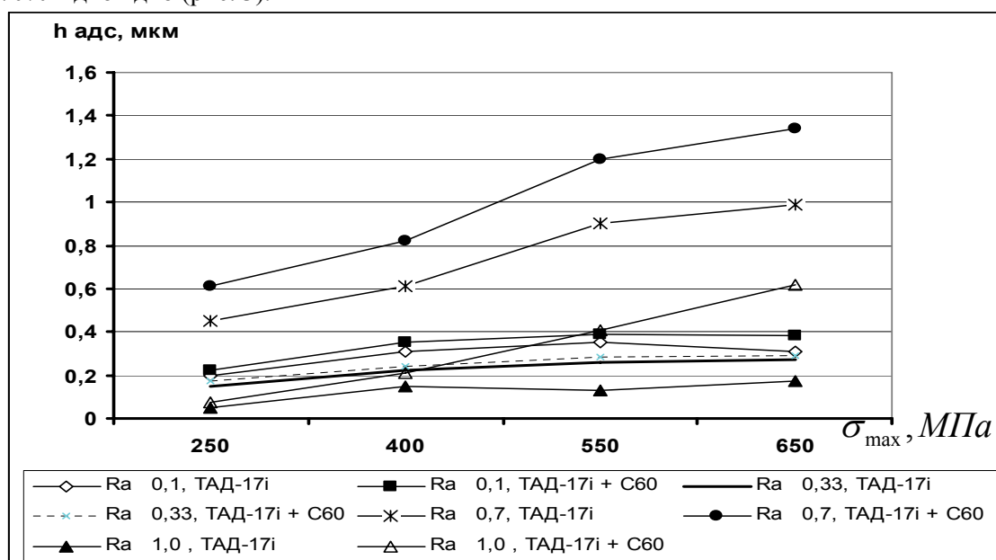
Рисунок 3 – Кінетика утворення граничних змащувальних шарів при збільшенні навантаження
