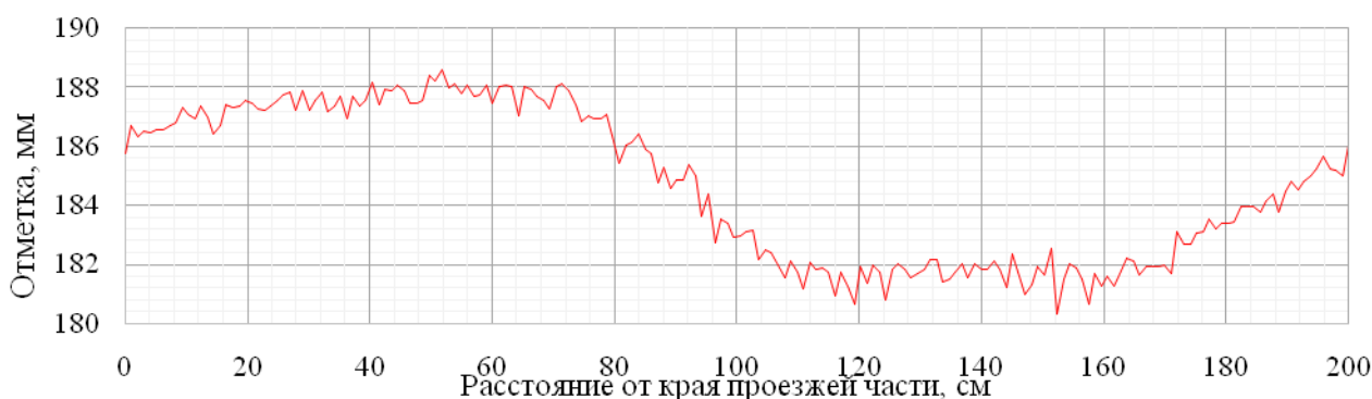
Рисунок 22– Пример записи результатов сканирования профиля поверхности дорожного покрытия
