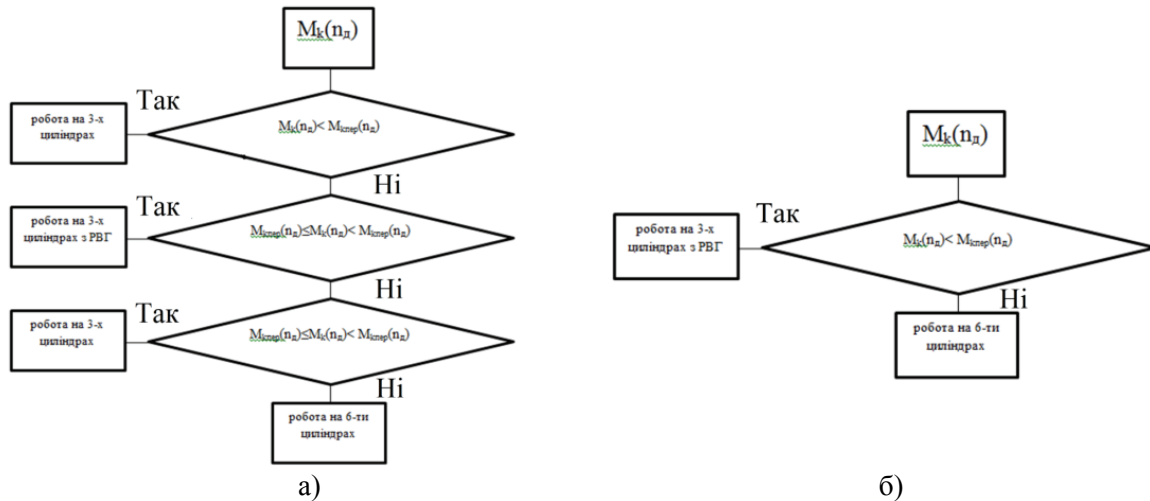
Рисунок 4 - Алгоритми розрахунку на математичній моделі руху транспортного засобу за режимами Європейського їздового циклу, які враховують моменти переключення з 6-ти циліндрів на 3-ти циліндри, і навпаки: а) отримання найкращої паливної економічності; б) отримання покращених екологічних показників.
