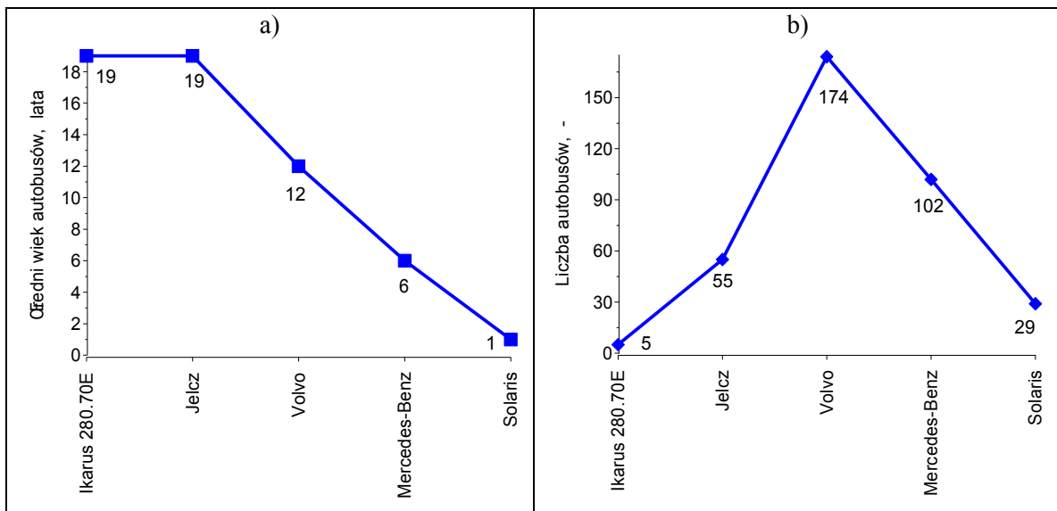
Rys. 1. Charakterystyka eksploatacyjna autobusów w MPK Wrocław: a) średni wiek, b) liczba autobusów w grupie
