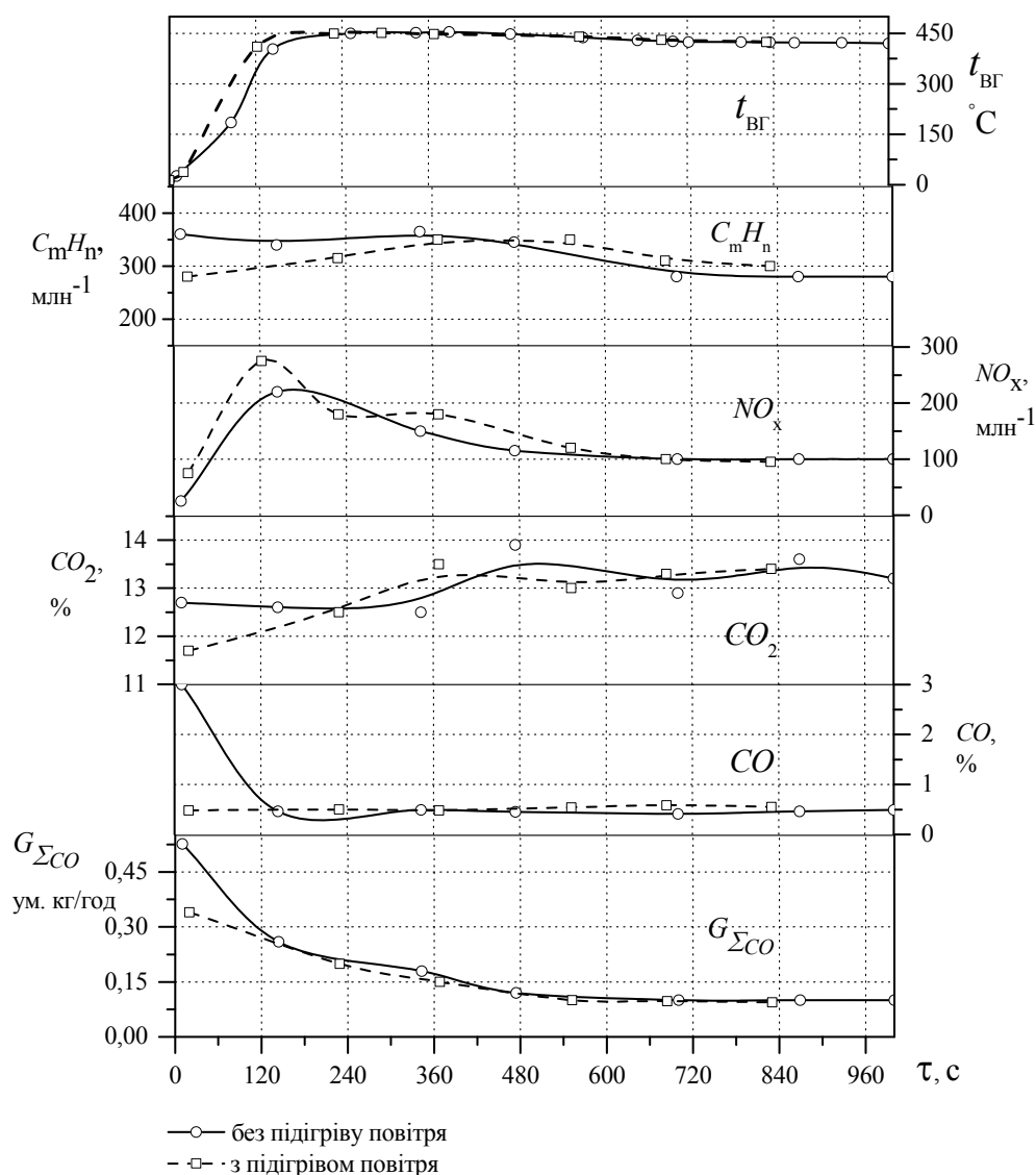
Рисунок 2 – Зміна концентрацій шкідливих речовин у ВГ двигуна до попереднього блока трикомпонентного каталітичного нейтралізатора в режимі прогріву
