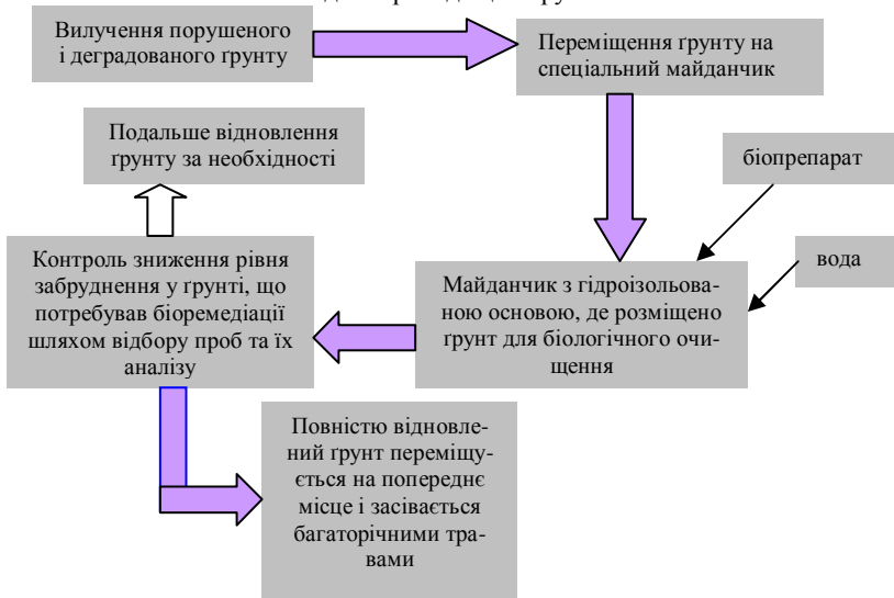
Рис. 2. Схема очищення ґрунту на гідроізолювальному рекультиваційному майданчику
