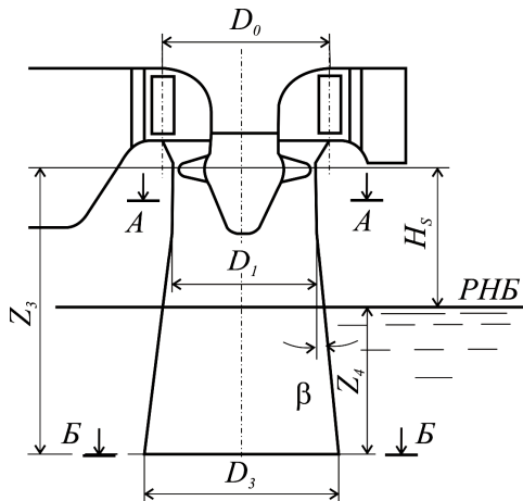
Рис. 1. Схема відсмоктувальної труби
