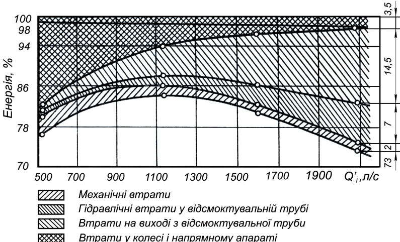
Рис. 2. Баланс енергії на моделі турбіни ПЛ
