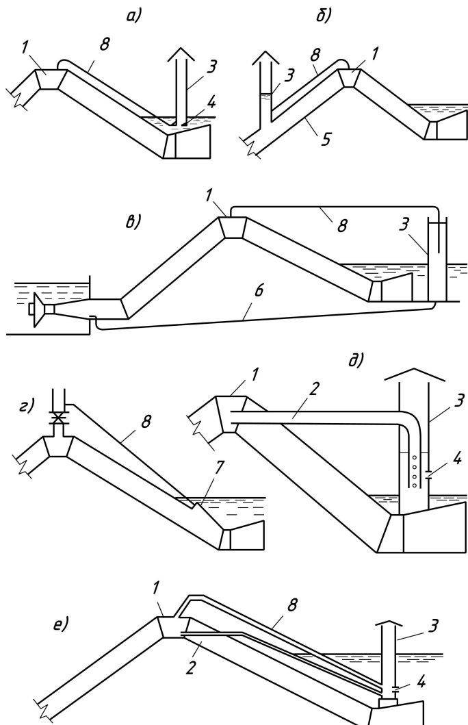
Рис. 1. Схеми гідравлічних клапанів зливу вакууму: 1 – сифон; 2 – швидкісна трубка; 3 – стакан; 4 – отвір; 5 – висхідна гілка; 6 – з'єднувальна трубка; 7 – кишень; 8 – повітропровід
