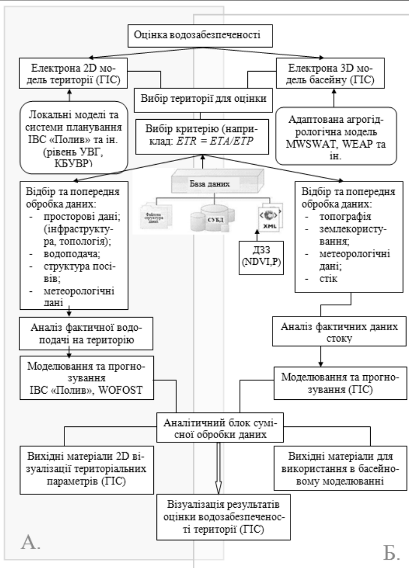
Рис. 1. Блок-схема балансової моделі системи оцінки наявного водоресурсного потенціалу території
