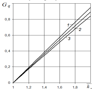
Рис. 1. Зависимость G_q(\bar{k}_u) : 1 – \bar{K}_I = -0.001 , 2 – \bar{K}_I = 0.001 , 3 – \bar{K}_I = 0.005
