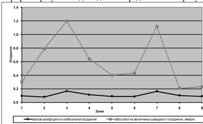
Рисунок. Зміни вагових коефіцієнтів небезпеки осідання та швидкості осідання за зонами
