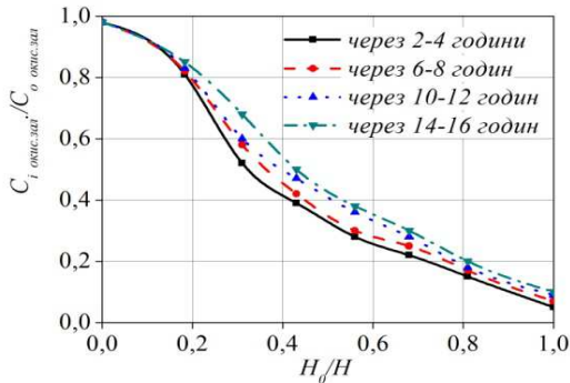
Рис. 3. Графік залежності зміни окисного заліза по висоті фільтруючого шару пінополістиролу ( V = 6,0 м/год, d = 1,25 мм, H = 1,2 м, C_{ок.зал.} = 3,5 мг/дм 3 , перманганатна окиснюваність 35 мг O_2/дм^3 , фільтроцикл № 10...12)
