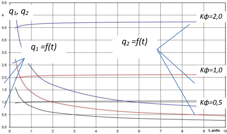
Рис. 3. Динаміка зміни в часі складових стоку з дрена ДЕМ
