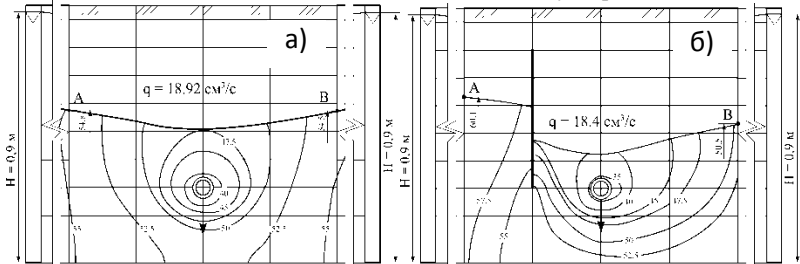
Рис. 4. Розподіл напорів навколо дрена при ґрунтовому живленні та рівних напорах в лотках: а – без екрана; б – з екраном
