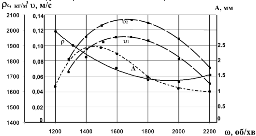
Рис. 1. Залежність густини середовища, швидкості спливання бурштину, амплітуди інтенсифікатора від частоти вібрації при експериментальних дослідженнях (A – амплітуда коливань вібронаряда; \rho – густина середовища; v_1 – швидкість спливання бурштину при подачі повітря q_{п} = 0,004 \text{ м}^3/\text{год.} ; v_2 – швидкість спливання бурштину при подачі повітря q_{п} = 0,006 \text{ м}^3/\text{год.} )
