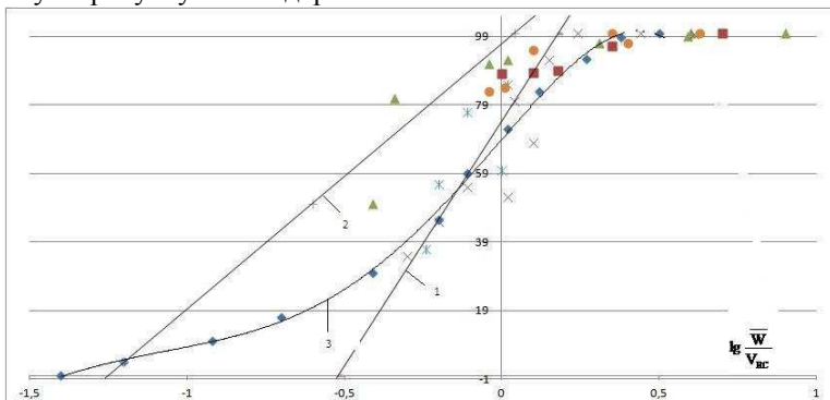
Рис. 6. Залежність процента захвату наносів в умовах від безрозмірної гідравлічної крупності наносів
