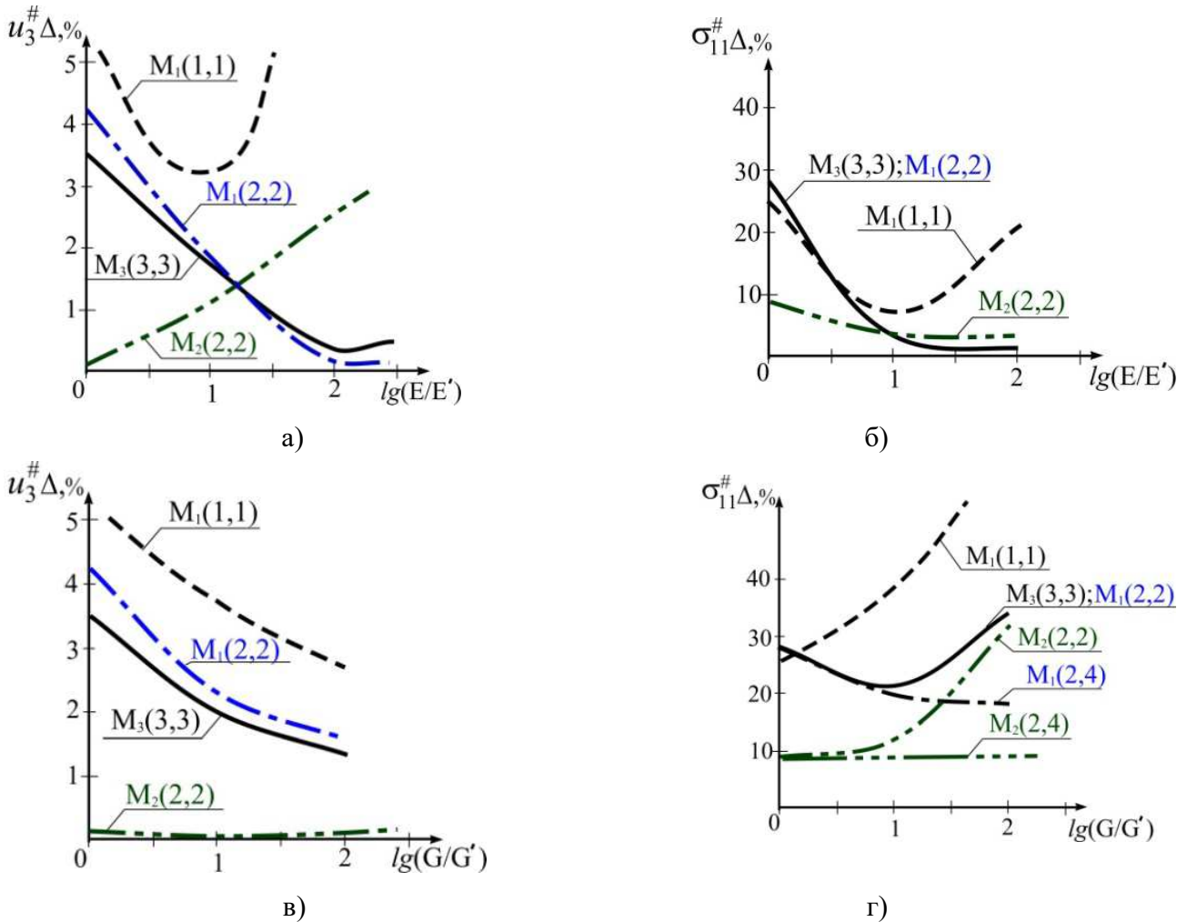
Рис. 3. Розподіл відносних похибок в однорідній транслопній плиті: а), в) для нормальних зміщень u_3^{\#} ; б), г) для максимальних напруг \sigma_{11}^{\#}
