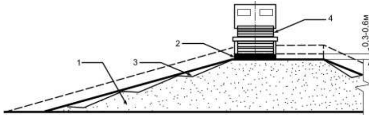
Рис. 8. Схема пошарового ущільнення ґрунтосуміші на гребені дамби: 1 – дамба; 2 – шар ущільнення ґрунтосуміші на гребені дамби; 3 – уступи; 4 – коток
