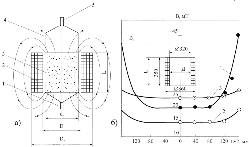
Рис. 1. Характер розподілу магнітного поля фільтра соленоїдного типу: а) вхідний 1 і вихідний 5 патрубкі; 2 – соленоїд; 3 – фільтруюча загрузка; 4 – корпус; б) розподіл поля в радіальному напрямку об'єму соленоїда: 1 – в торцевій площині з кульковою загрузкою ( B_p – розрахункова індукція в довгому соленоїді з еквівалентною кількістю витків на одиницю довжи- ни); 2 – в торцевій площині без загрузки; 3 – посередині соленоїда
