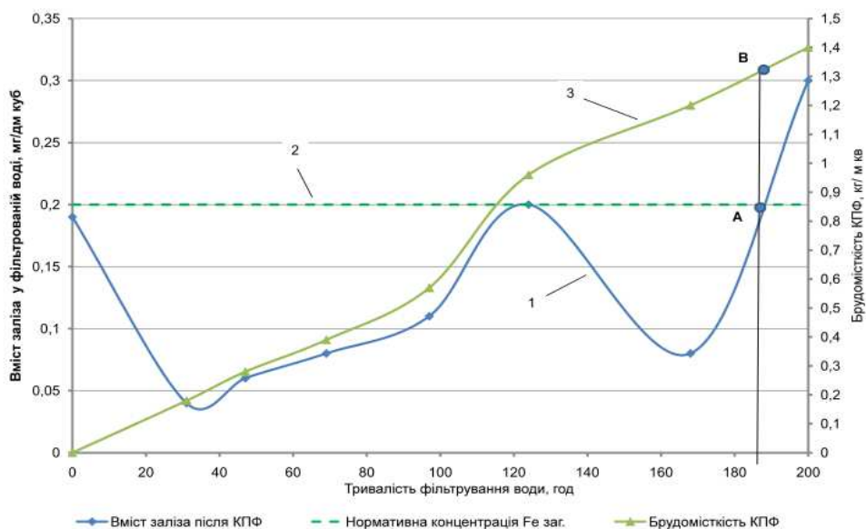
Рис. 3. Показники роботи КПФ протягом фільтроциклу: 1 – вміст заліза у фільтрованій воді, мг/дм 3 ; 2 – нормативний вміст заліза у питній воді ( C_n=0,2 мг/дм 3 ); величина брудомісткості КПФ, кг/м 2
