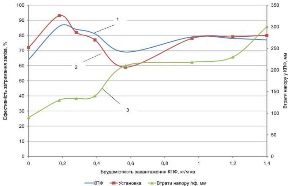
Рис. 4. Залежності ефективності очищення води E і втрат напору h_f від питомої брудомісткості фільтрувального завантаження: 1 – E=f(G_\phi) на КПФ; 2 – E=f(G_\phi) на установці; 3 – h_f=f(G_\phi)
