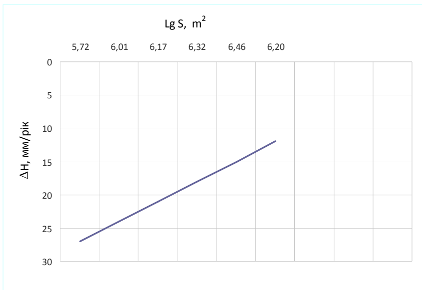
Рис. 4. Плоско-радіальний розвиток карстової деформації донної поверхні зони впливу поля шахти № 7
