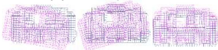
Рис.10. Формы колебаний частичных систем 2-го уровня перекрытия здания по ул. Проценко ,50
