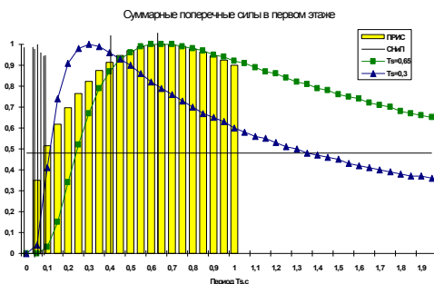
Рис. 6 Зависимость поперечных сил от преобладающих периодов T_s сейсмических волн
