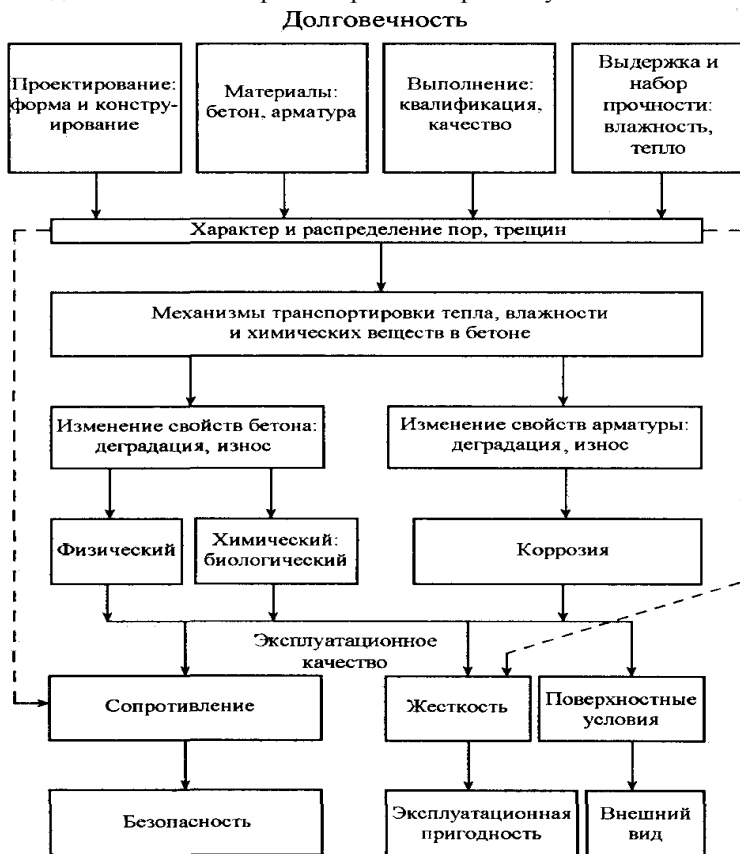
Рис. 2. Соотношение между долговечностью железобетонных конструкций и их эксплуатационным качеством
