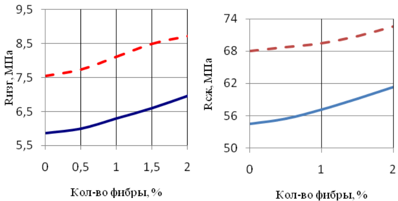
Рис. 1. Влияние количества базальтовой фибры на прочность базальтоцемента
