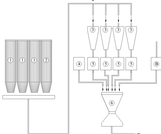
Рис.2. Технологическая схема производства механоактивированных композиций на основе минеральных вяжущих
