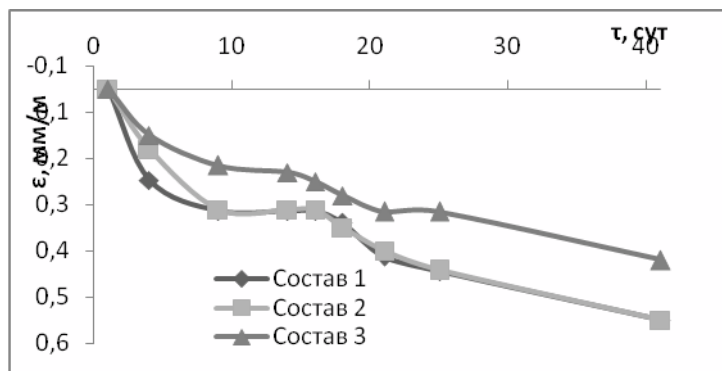
Рис. 3. Кинетика изменения усадочных деформаций контрольного газобетона (состав 1) и модифицированного микрофиброй 900 \text{ г} / \text{м}^3 и 500 \text{ г} / \text{м}^3 газобетонов (состав 2 и 3) соответственно.
