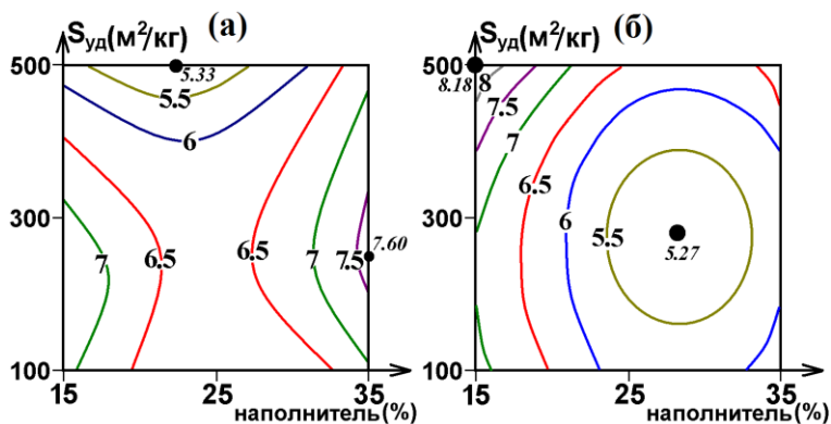
Рис.2. Влияние наполнителя и внешних воздействий на конец схватывания цементных композиций.
