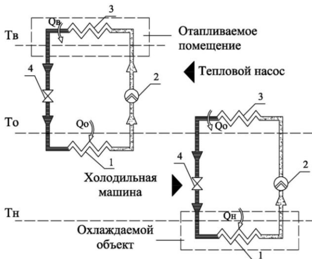
Рис.1. Схема и условия трансформации теплоты в системе «Охлаждаемый объект – отапливаемое помещение». Условные обозначения: 1 – испаритель; 2 – компрессор; 3 – конденсатор; 4 – дроссельный вентиль
