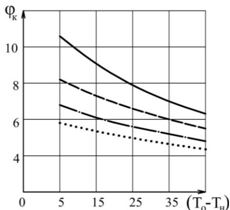
Рис.2. Зависимость коэффициента преобразования по циклу Карно в термотрансформаторной системе теплохладоснабжения от (T_0 - T_n) и T_b .
