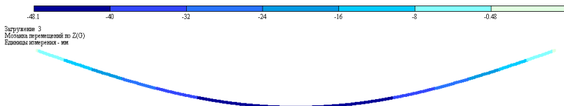
Рис.12. Мозаика перемещений балки
