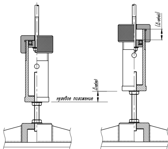
Рис. 4. Установка предварительной слабину
