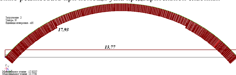
Рис.7. Эпюра продольных сил в арке
