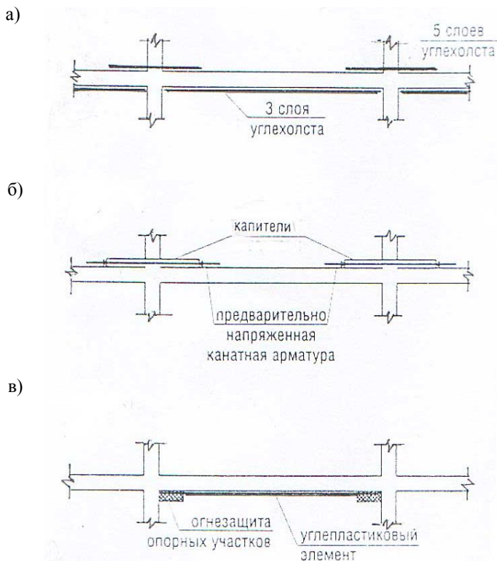
Рис. 2. Схема комбинированного усиления 9-метровых ригелей железобетонных перекрытий многоэтажного здания: а) наклейкой углепластика; б) с изменением расчетной схемы путем устройства капителей, расположенных на перекрытии, с последующим выполнением их локального предварительного напряжения, а в зоне действия пролетных моментов наклеивали углеродный холст; в) компенсирование приращения изгибающего момента в пролете путем устройства внешнего армирования из углепластика
