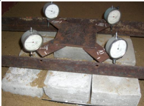
Рис. 2. Индикаторы часового типа для определения осадки образца
