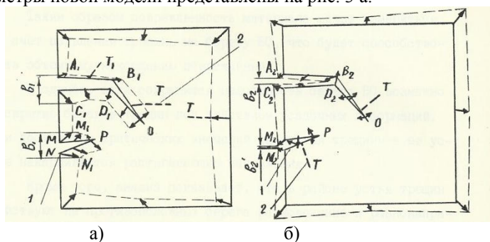
Рис. 3. Распределение деформаций усадки (а) и набухания (б) в модели бетона с K_p = 0,15:1 – начальная трещина; 2 – эксплуатационные трещины; v_1, v_1 – ширина раскрытия трещины; v_2, v_2 – ширина смыкания трещины
