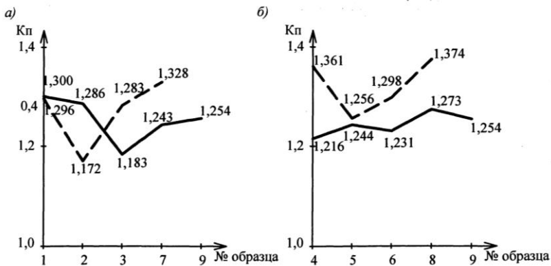
Рис. 2. Изменение коэффициента поврежденности в зависимости от формы заполнителей при кубической (а) и гексагональной (б) упаковке (грани 40х90мм):
