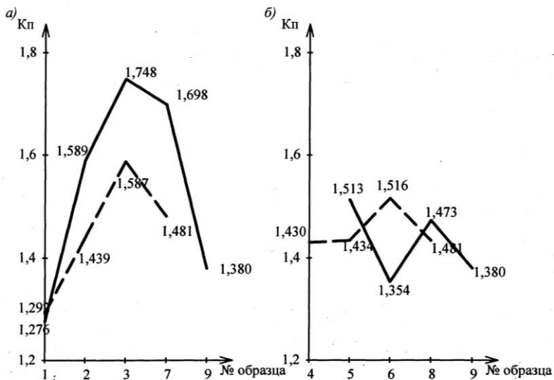
Рис. 3. Изменение коэффициента поврежденности в зависимости от формы заполнителей при кубической (а) и гексагональной (б) упаковке (грани 40х160 мм):
