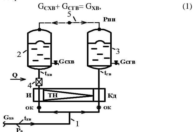
Рис. 2. Схема к определению условий пневмогидравлической стабилизации движения водных потоков через конденсатор и испаритель теплонаносной установки. Условные обозначения: 1 – тру-бопровод холодной воды; 2 – бак – аккумулятор холодной воды; 3 – бак – аккумулятор горячей воды; 4 – калорифер системы воздушного охлаждения здания; 5 – трубопровод, соединяющий надмембранные части баков – аккумуляторов; И – испаритель; КД – конденсатор; ОК – обратный клапан
