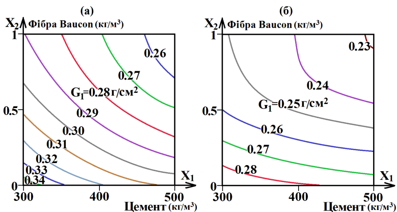
Рис.3. Вплив варійованих факторів складу на стиранність бетону. а – склади на гранітному щебені, б – склади на карбонатному щебені
