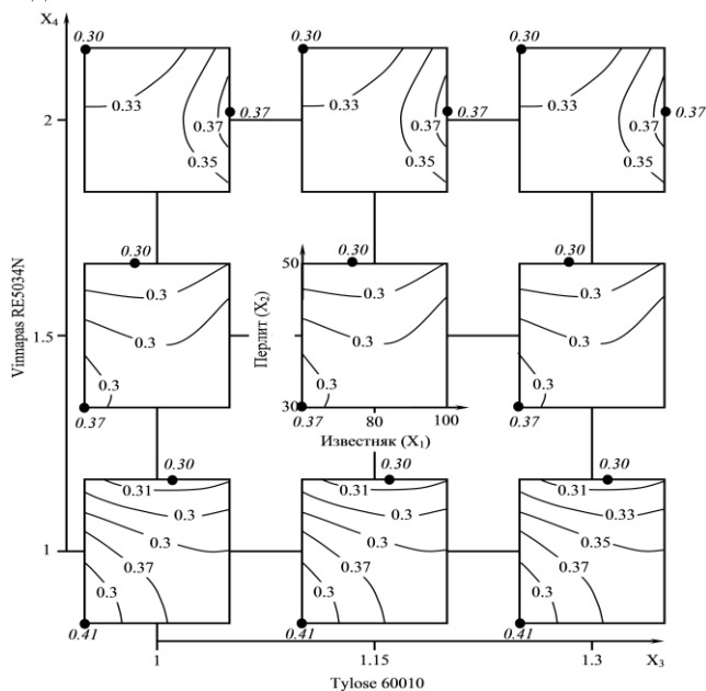
Рис. 2. Влияние варьируемых факторов состава теплопроводность, Вт/м·К
