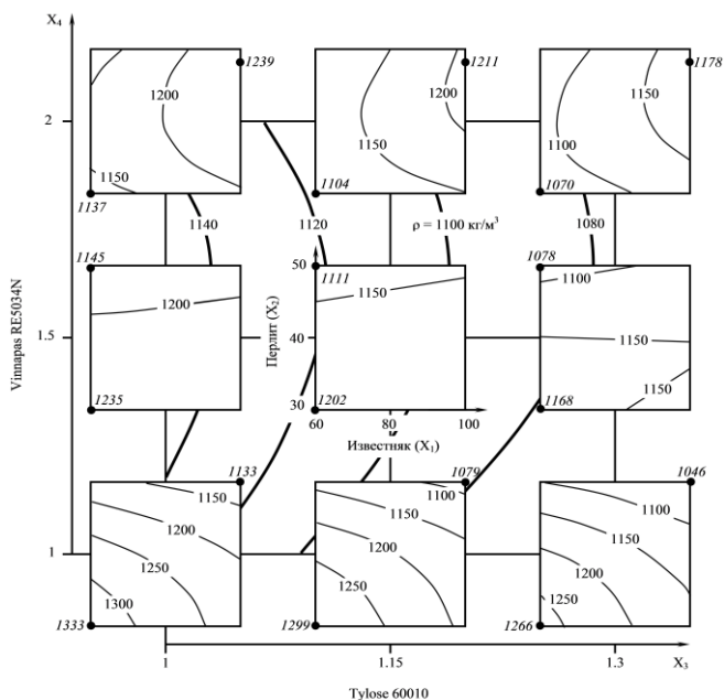
Рис.1. Влияние варьируемых факторов состава на плотность затвердевшего раствора ( \text{кг}/\text{м}^3 )
